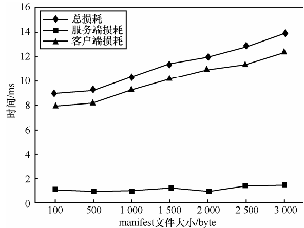
图 9 Sec-Cache 方案损失时间
